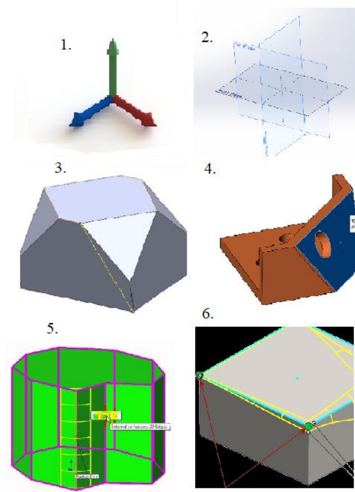
Slika 4. SolidWorks modeli [4].
