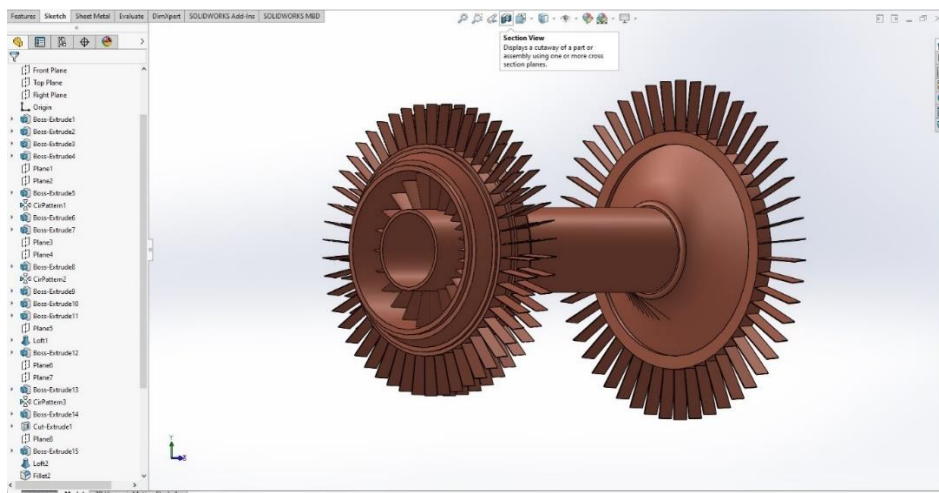
Slika 33. Model osovine 02
