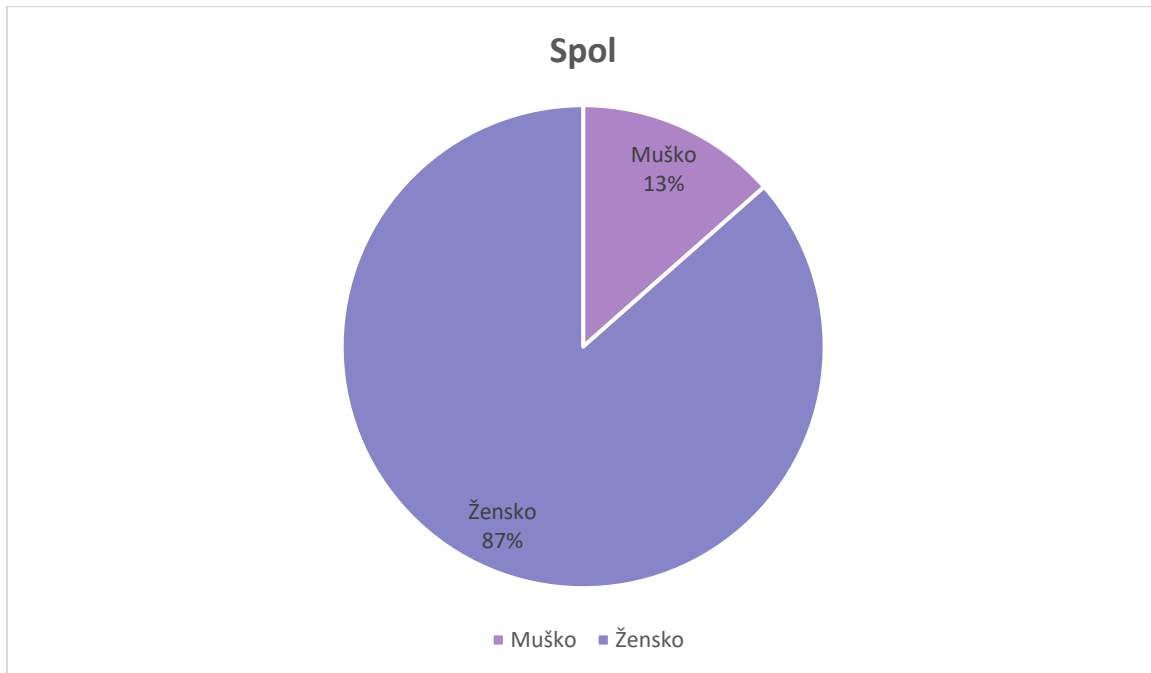
Grafikon 1. Spol
