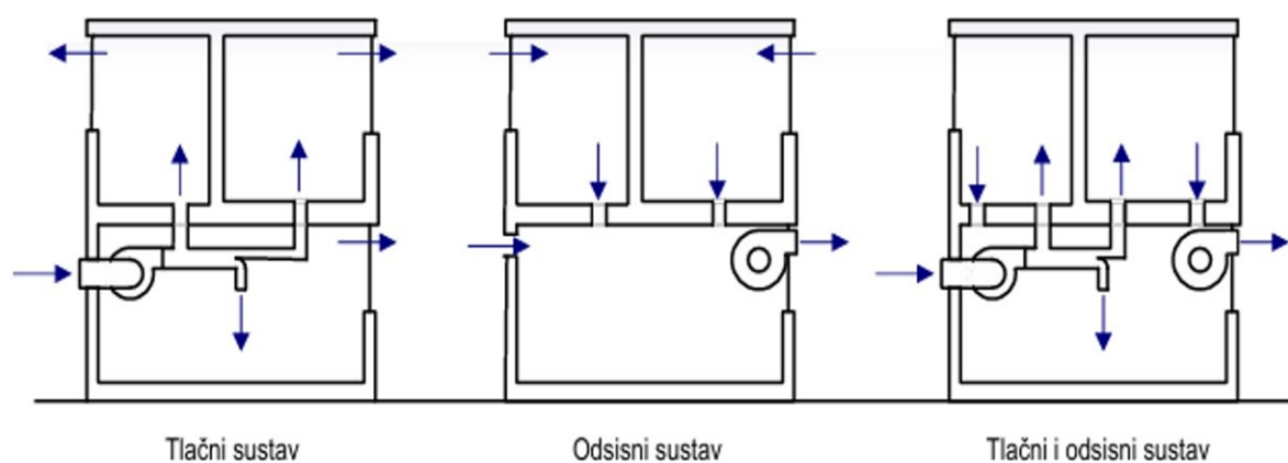
Slika 4. Pojednostavljeni prikaz sustava ventilacije prema tlaku u prostoru [1]
