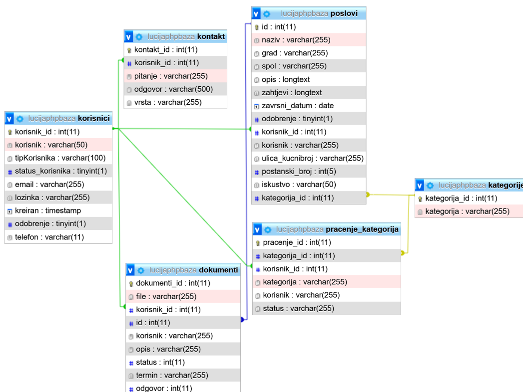
Slika 2. ER model
