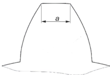
Slika 19 Evolventni profil zuba
