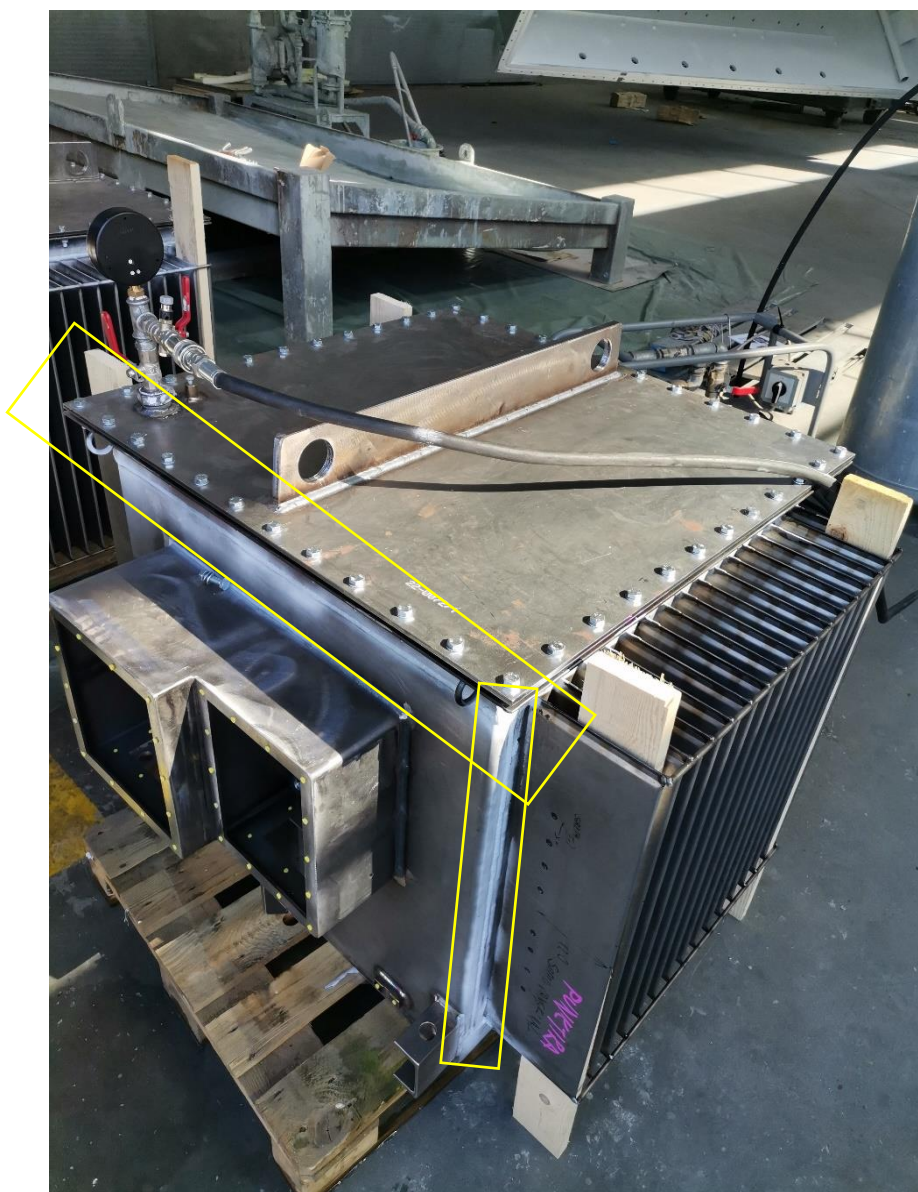
Slika 25. Nanos penetranta
