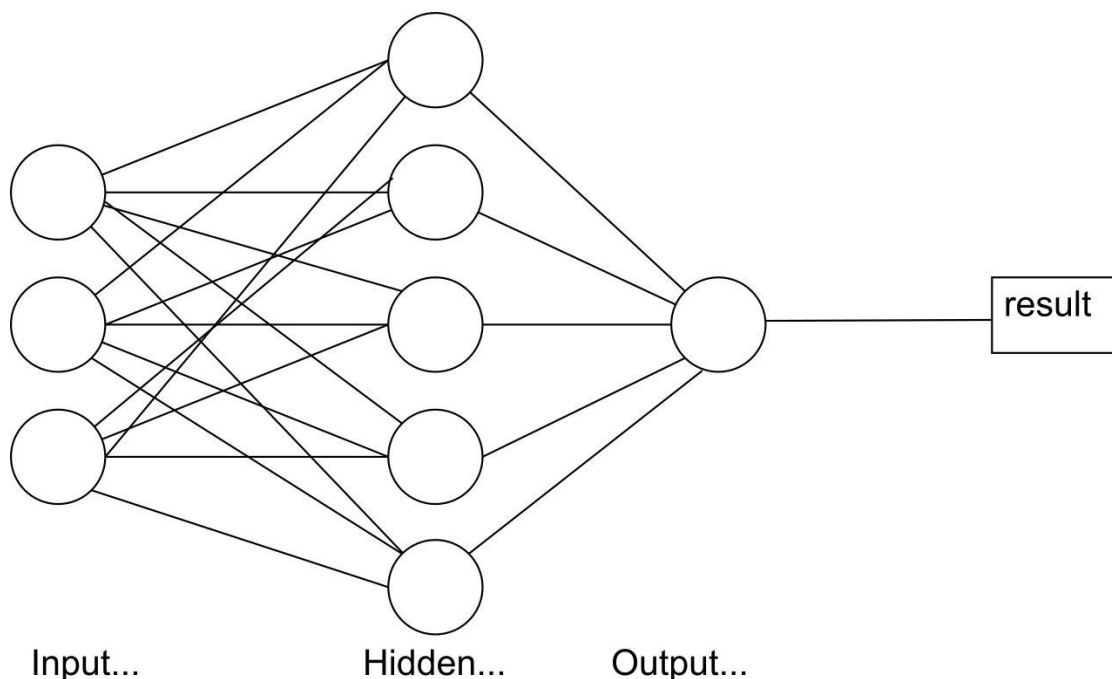
Slika 2. Struktura MLP-a
