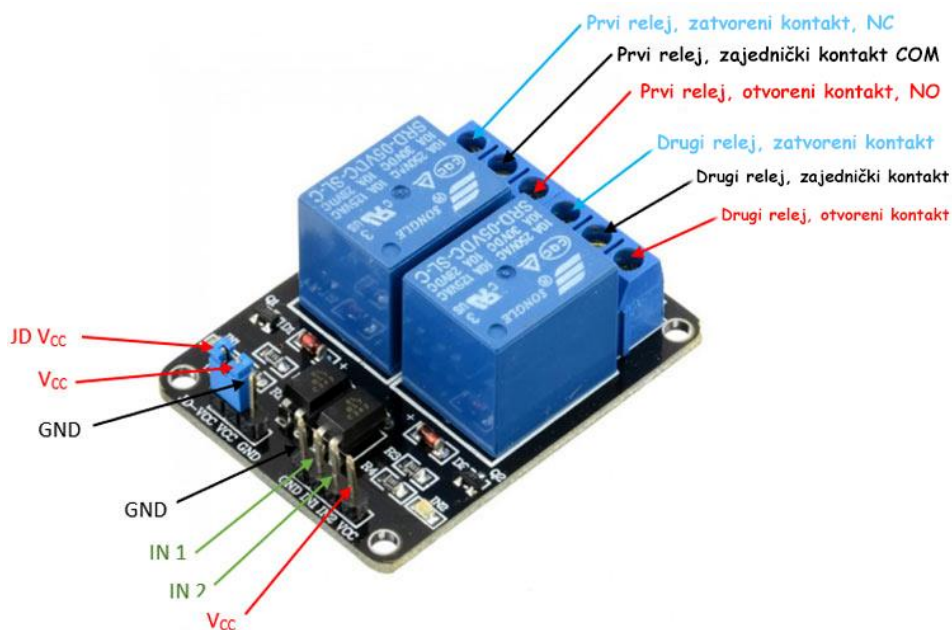
Slika 7. Relej JQC3F
