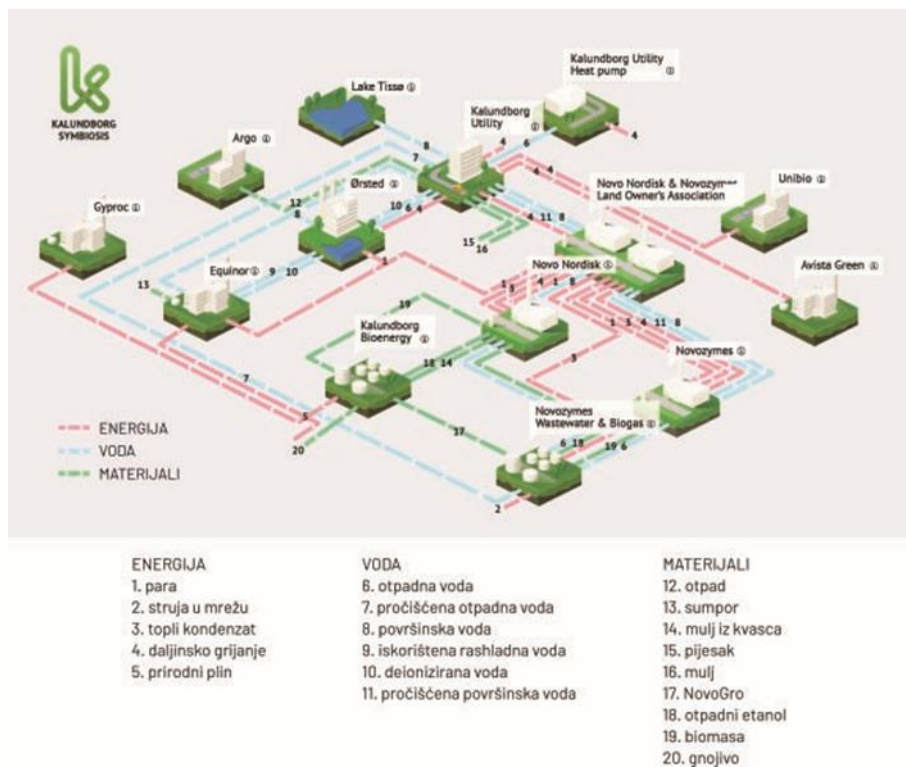
Slika 4: Kalundborg simbioza [28]
