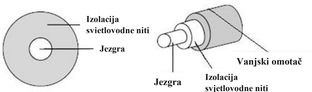
Slika 2. Presjek svjetlovodnog kabela (Izvor.
