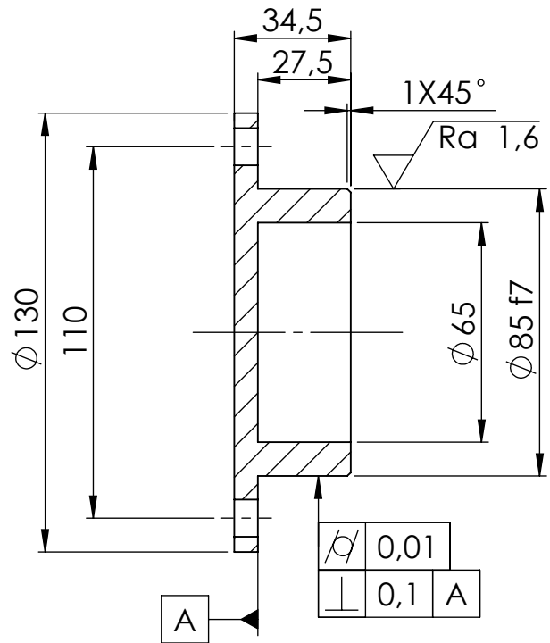
Presjek A-A
