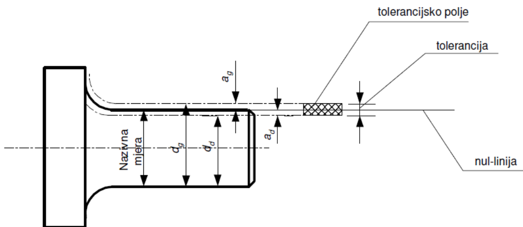
Slika 14 Prikaz tolerancija
