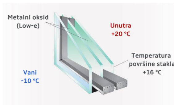
Slika 5. Prozor s niskoemisijjskim premazom
