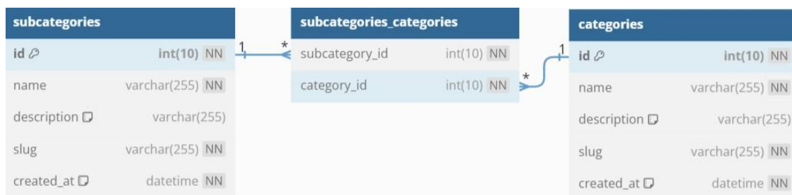
Slika 38. Tablica „subcategories_categories“ i veze s tablicama „subcategories“ i „categories“
