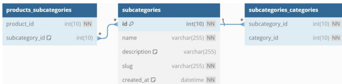
Slika 37. Tablica „subcategories“ i veze s tablicama „products_subcategories“ i „subcategories_categories“
