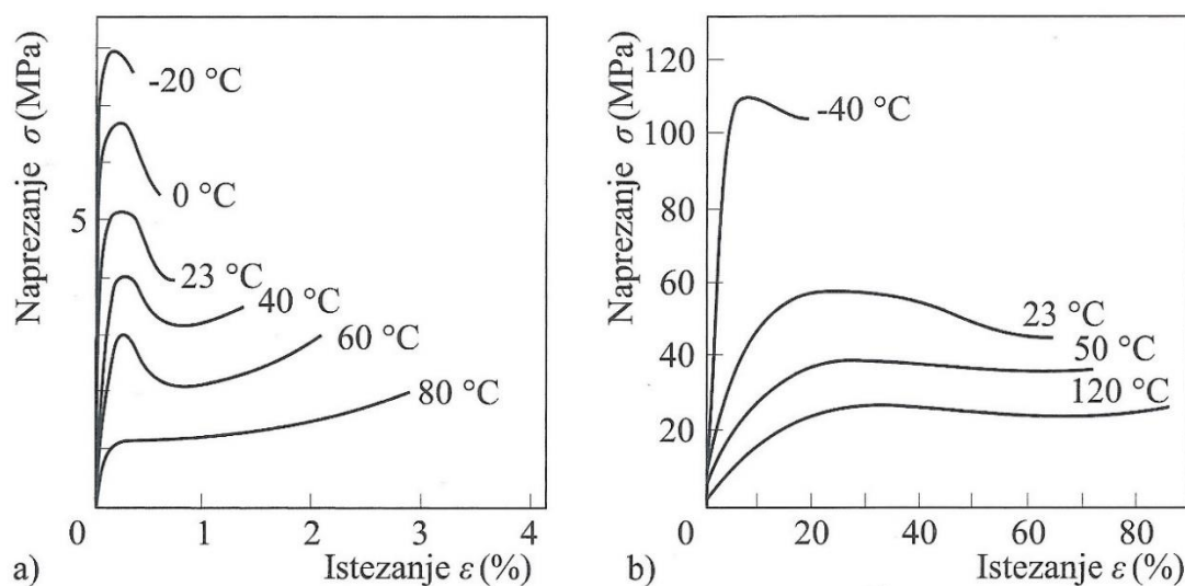
Slika 8. Utjecaj temperature na oblik krivulje ovisnosti napreznja i istezanja PVC-a (a) i PA66 (b)
