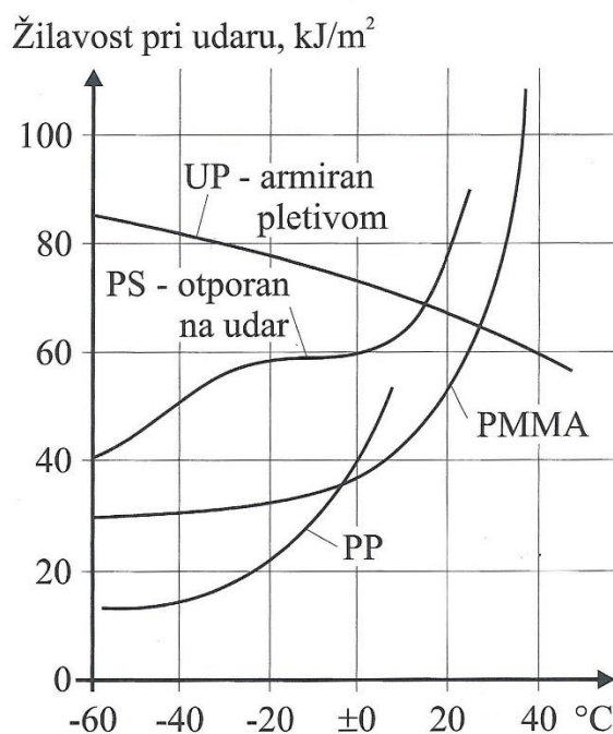
Slika 5. Žilavost u ovisnosti o temperaturi
