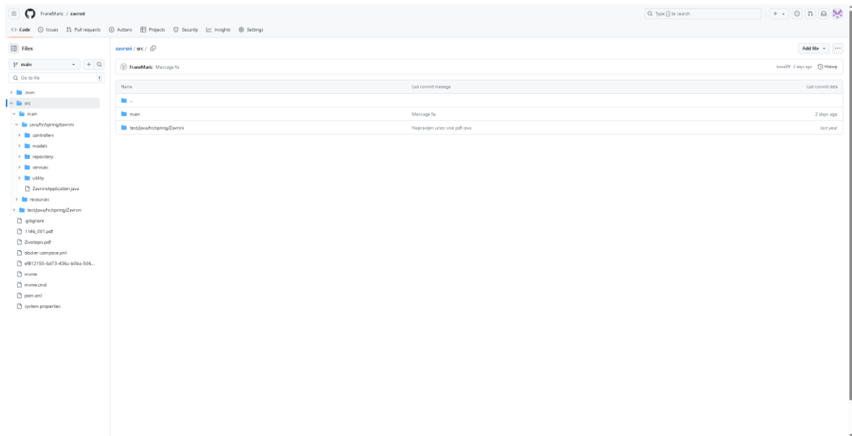
Slika 4. GitHub
