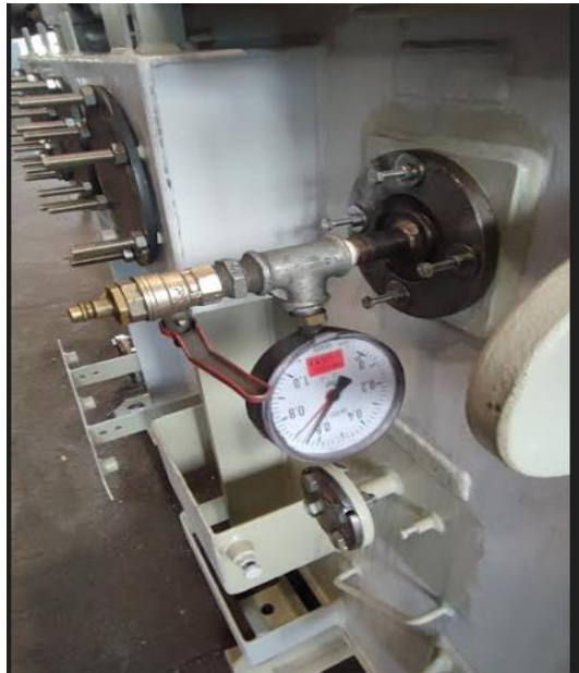
Slika 28. Zatvaranje kotla i postavljanje manometra
